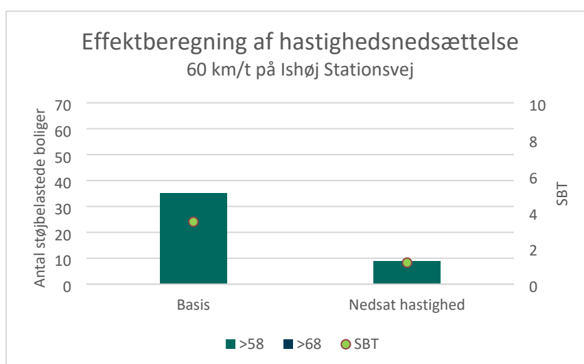
Figur 19: Effektberegning af en hastighedsnedsættelse til 60 km/t på Ishøj Stationsvej.
