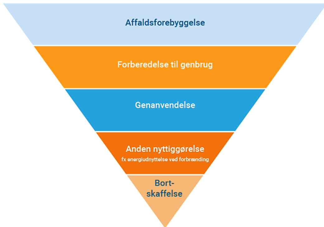
Figur: Affaldspyramiden
