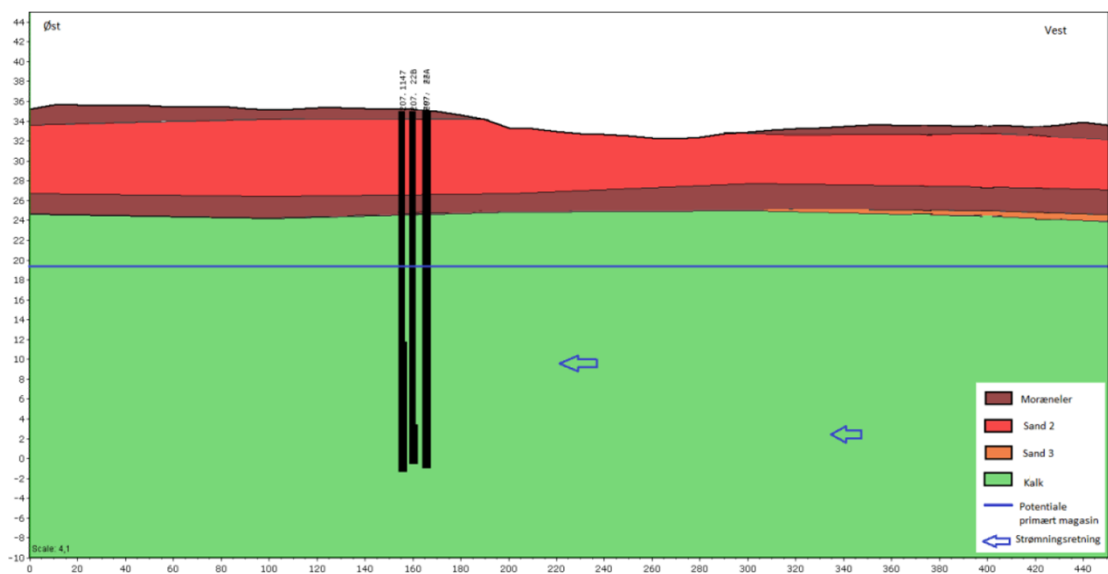
Figur 7-3. Geologi ved Hedehusene Østre Vandværk med angivelse af potentiale i det primære magasin.
