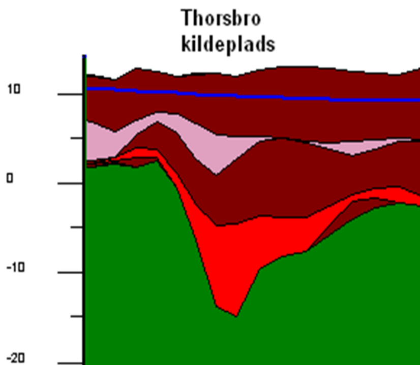
Figur 3-2 Geologi på Thorsbro kildeplads med angivelse af potentialeniveau i det primære magasin (blå streg). Kalken (grøn) overlejres af sand (rød og lyserød) og 7-15 meter ler (brun).
