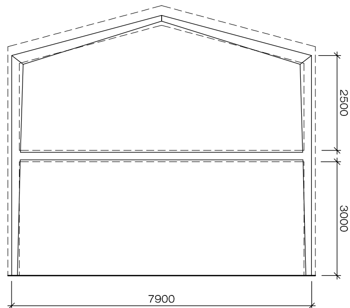
Principsnit - bygning med udnyttet tagetage, mål 1:100
