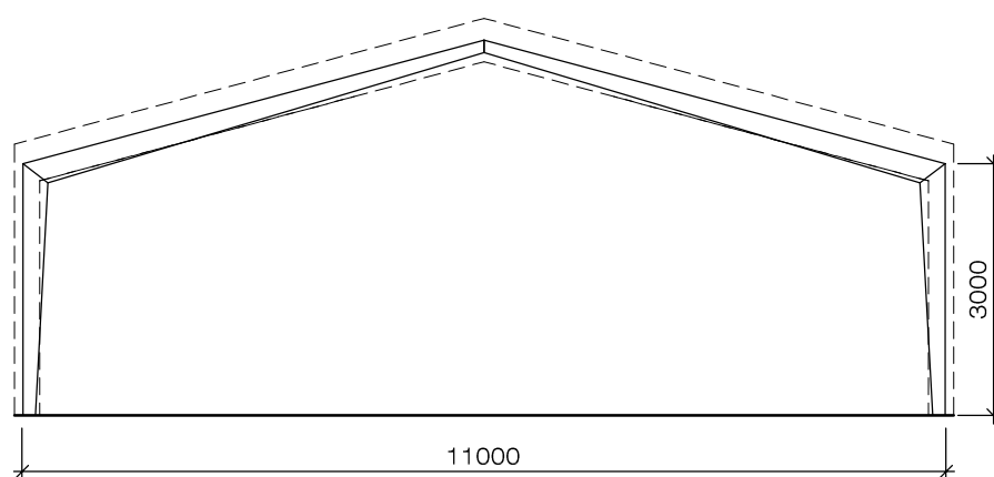
Principsnit - bygning i en etage, mål 1:100
