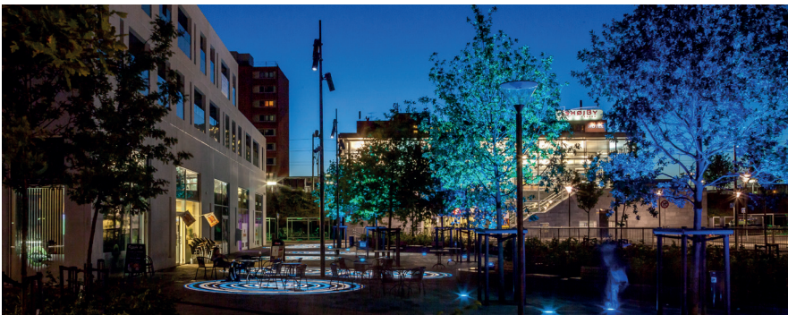
Lysudsmkning på Ishøj Stationsforplads.
