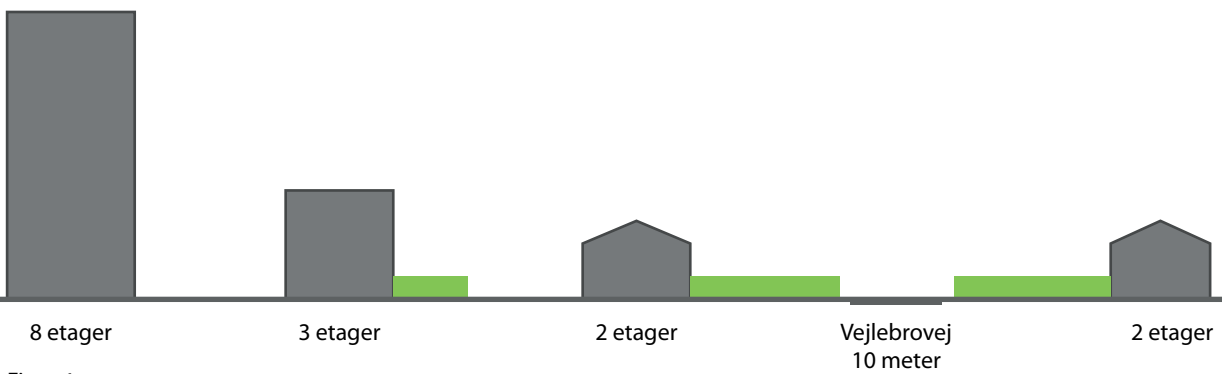
Figur 1 Tværsnit A-A over Vejlebrovej
