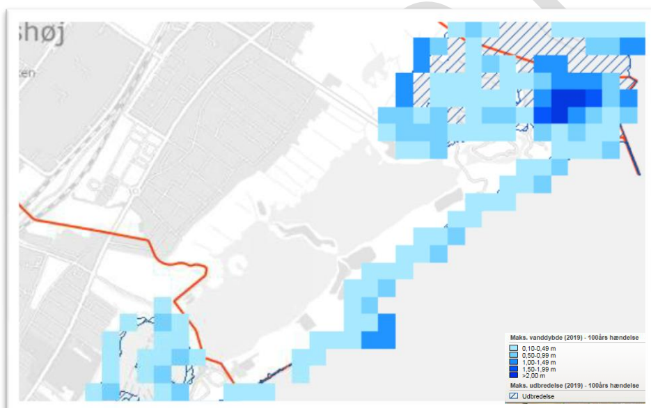
Figur 3 100 års stormflod i 2019 med en vandstand på 159 cm
