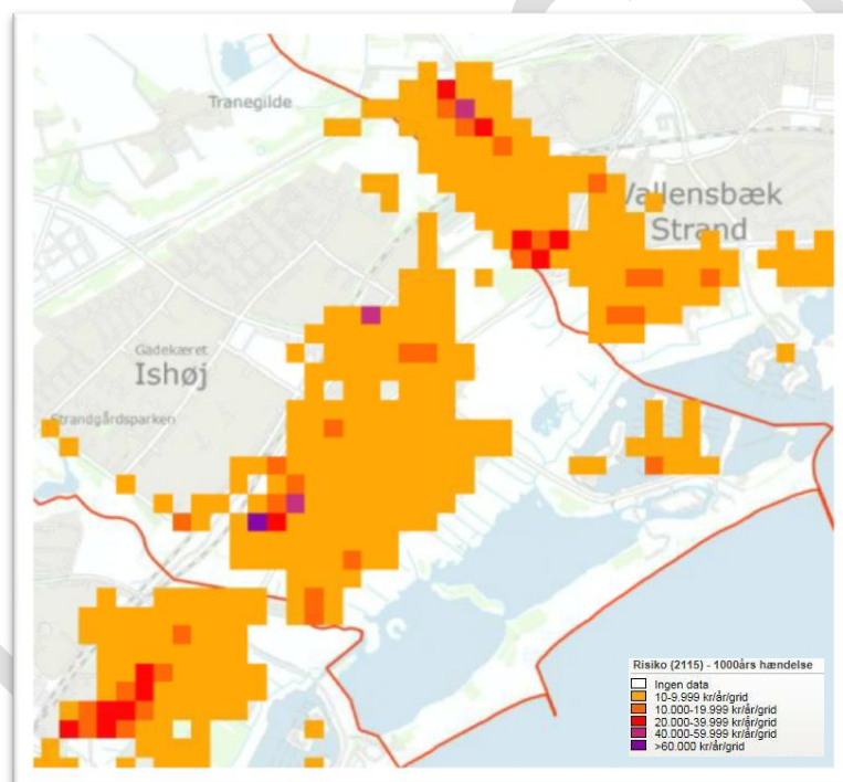
Figur 8 Risiko ved en ekstrem hændelse i 2115. Vandstand 3,48 m.
