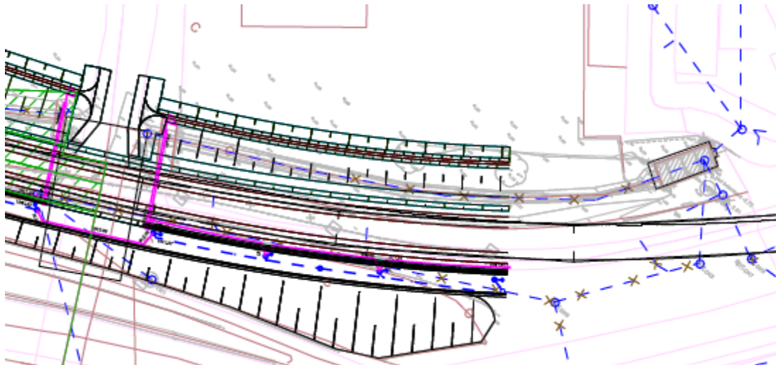
Figur 2. Tegningsudsnit over fremtidig grøft.
